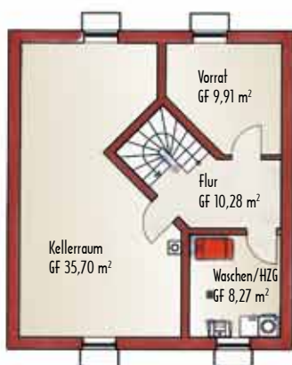
Kellergeschoss Maßstab 1:200
